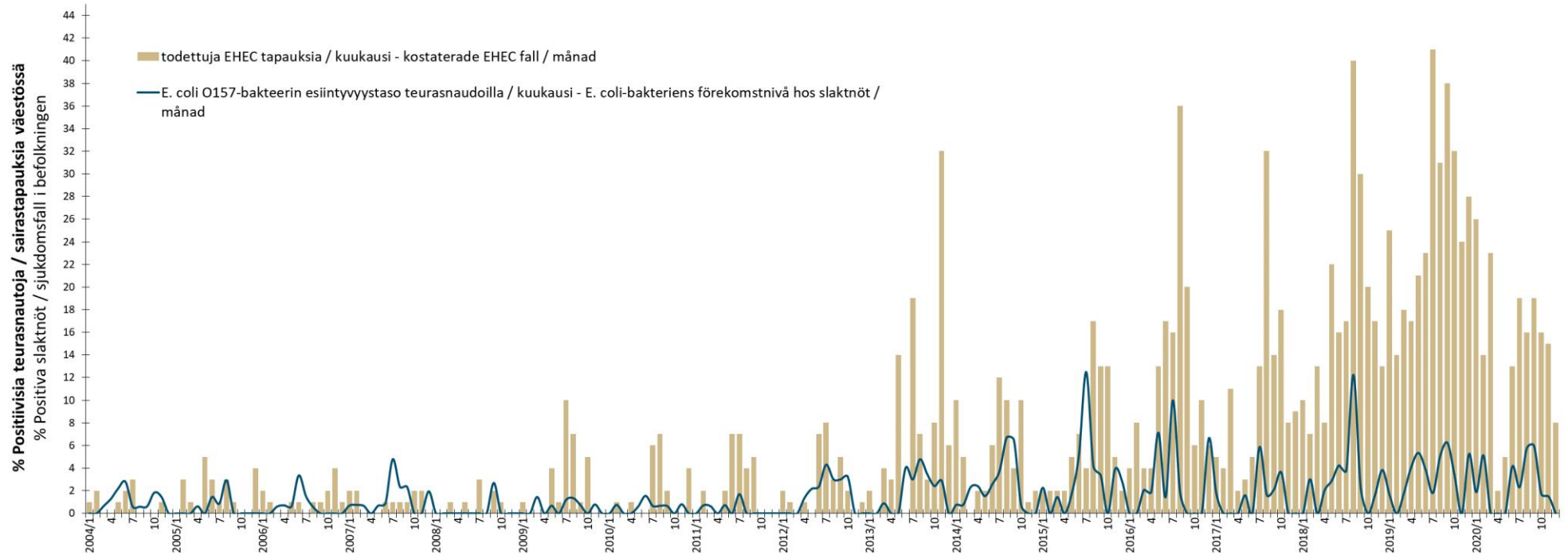
Kuva. E. coli O157 -bakteerin esiintyvyys teurasnaudoilla sekä EHEC sairastapaukset väestössä kuukausittain vuodesta 2004 (Lähteet: EHEC-valvontaohjelma, Evira (nykyinen Ruokavirasto); Tartuntatautirekisteri, THL)
