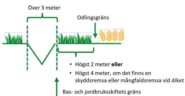
Bild 1: Mätning av kantdikets bredd.
