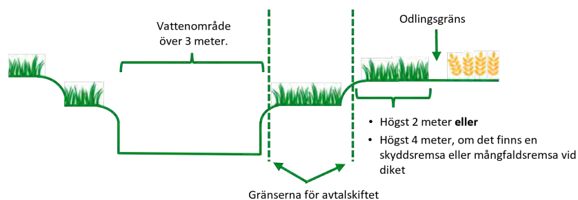
Bild 3. Tvåstegsdike med skötselavtal
