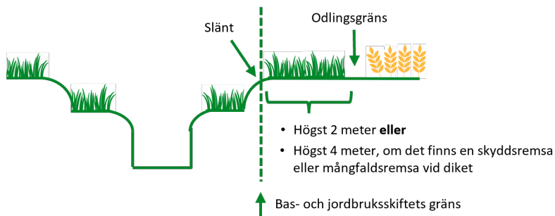
Bild 2. Tvåstegsdike
