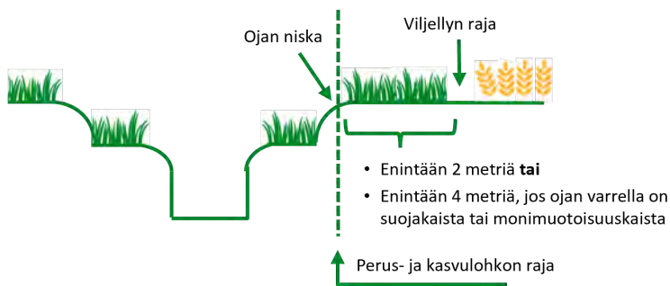
Kuva 2. Kaksitasouoma
